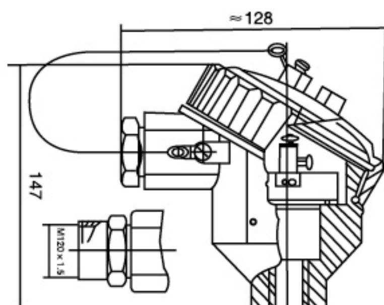
防水式接线盒
