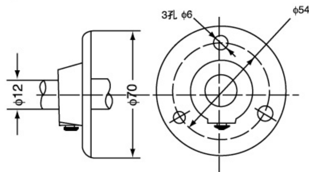
活动法兰式
