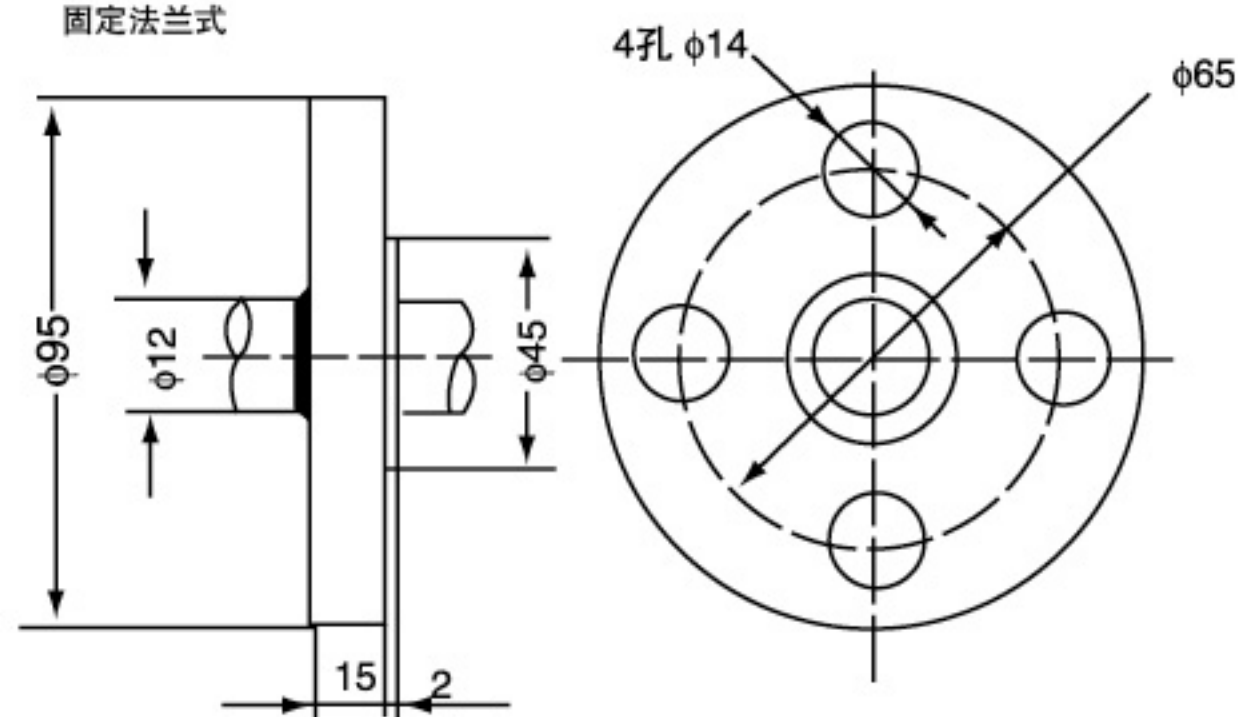
固定法兰式
