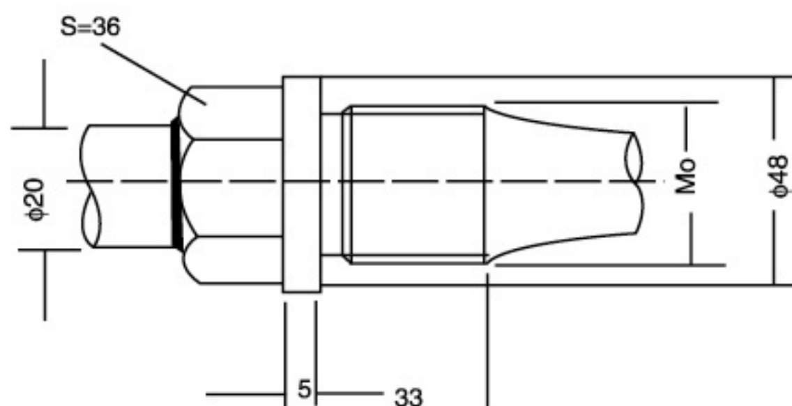
固定螺纹锥形保护管式
