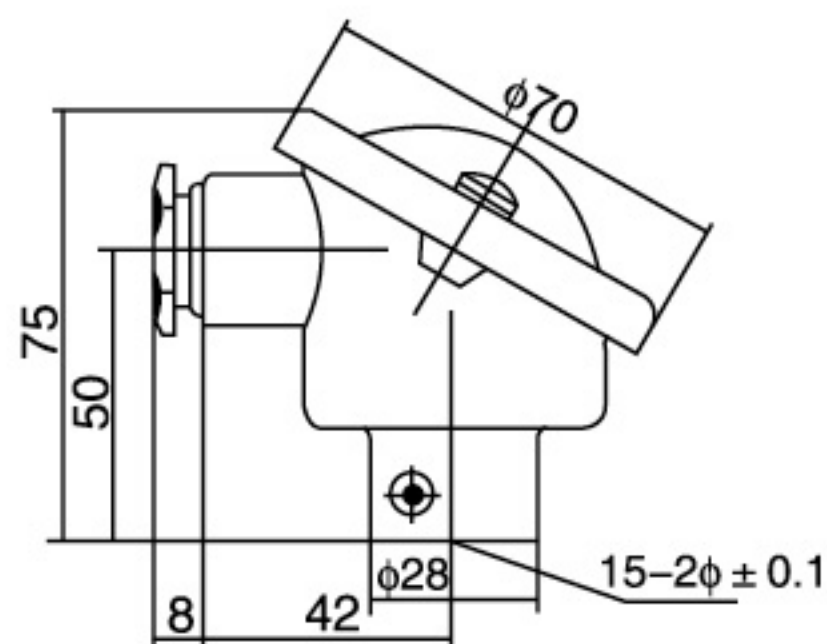
防溅式接线盒
